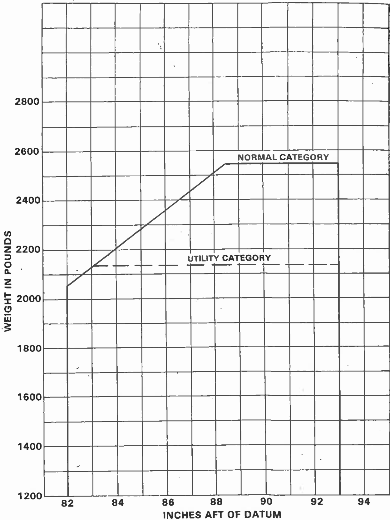
C. G. RANGE AND WEIGHT
